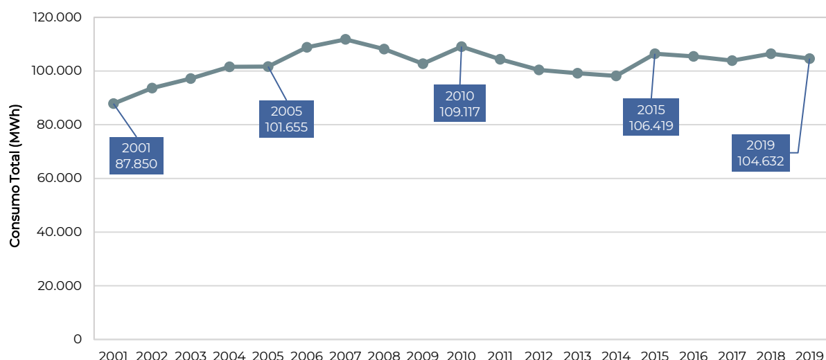
Gráfico 42: Consumo total de energia elétrica [MWh/ano], no território do concelho de Vale de Cambra, no período 2001-2019
