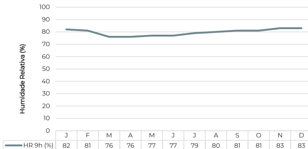
Gráfico 22: Humidade Média Relativa 9h (%)
